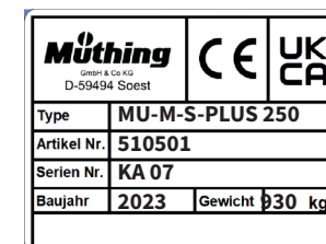
Beispiel Typenschild | Type plate example Exemple de plaque signalétique | Ejemplo de una placa de características
